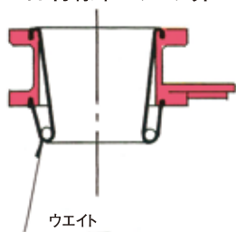
ウェイト付標準スリーブ弁
