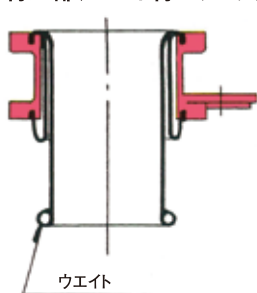
ウェイト付上部シュート付スリーブ弁
