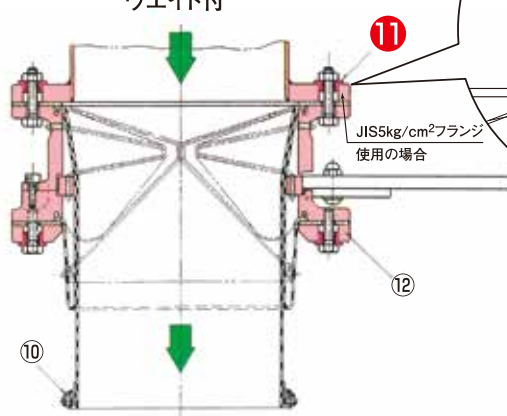
上部シュート付スリーブ弁 ウエイト付
